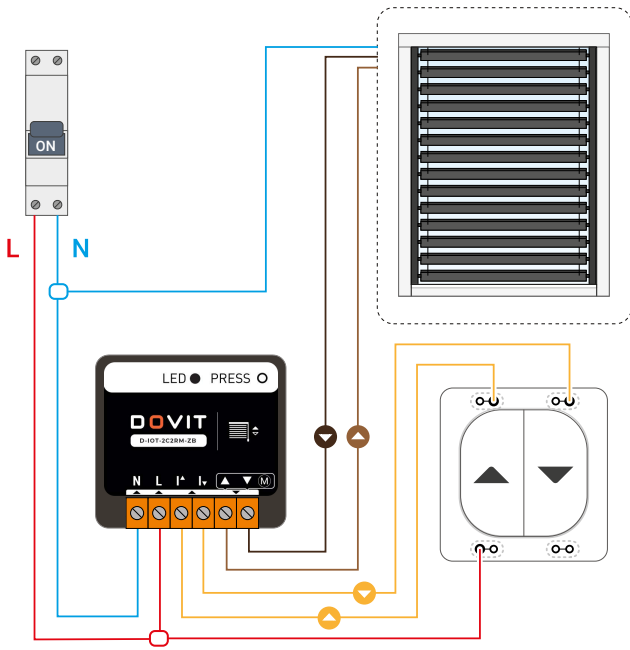
Rolling sunshades
